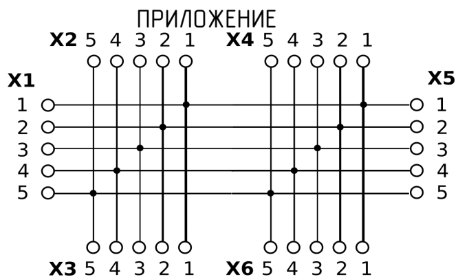
Рис. 1. Схема принципиальная ПР-6У.
